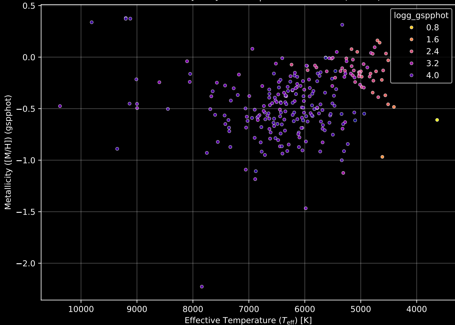
GALAH DR4 Field: [8823] Stellar Population Parameters (n= 258)
