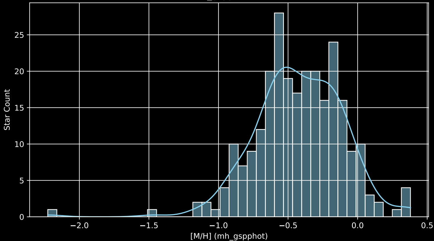
GALAH DR4 Field: [8823] [M/H] (mh_gspphot) (n= 258)
