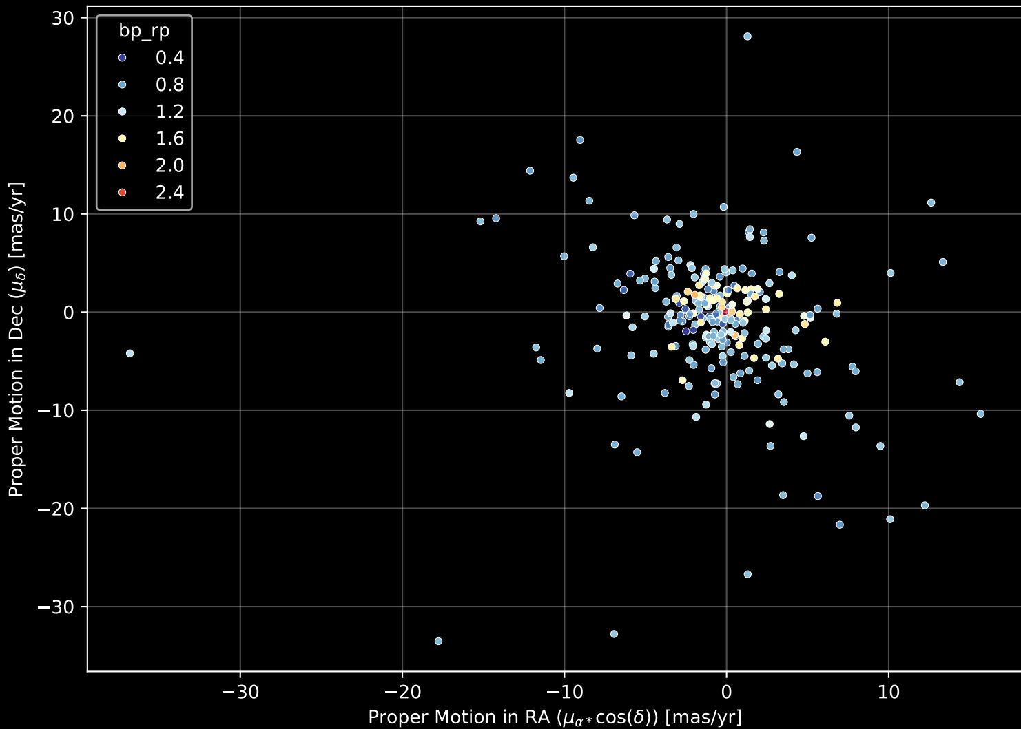
GALAH DR4 Field: [8823] Proper Motion Diagram (n= 258)
