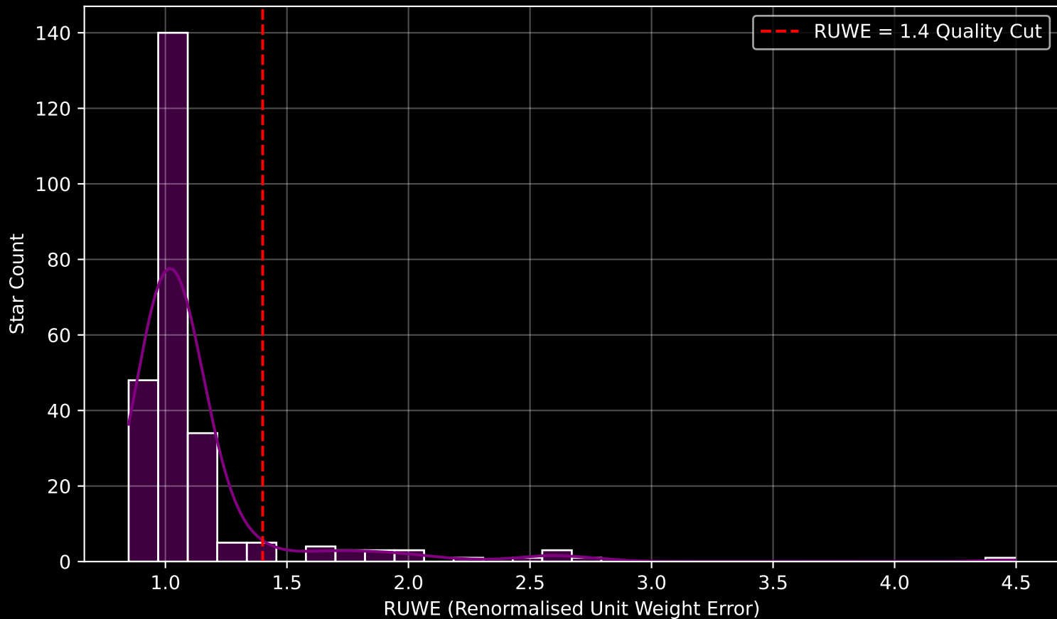
GALAH DR4 Field [8823] RUWE Distribution (n= 252)
