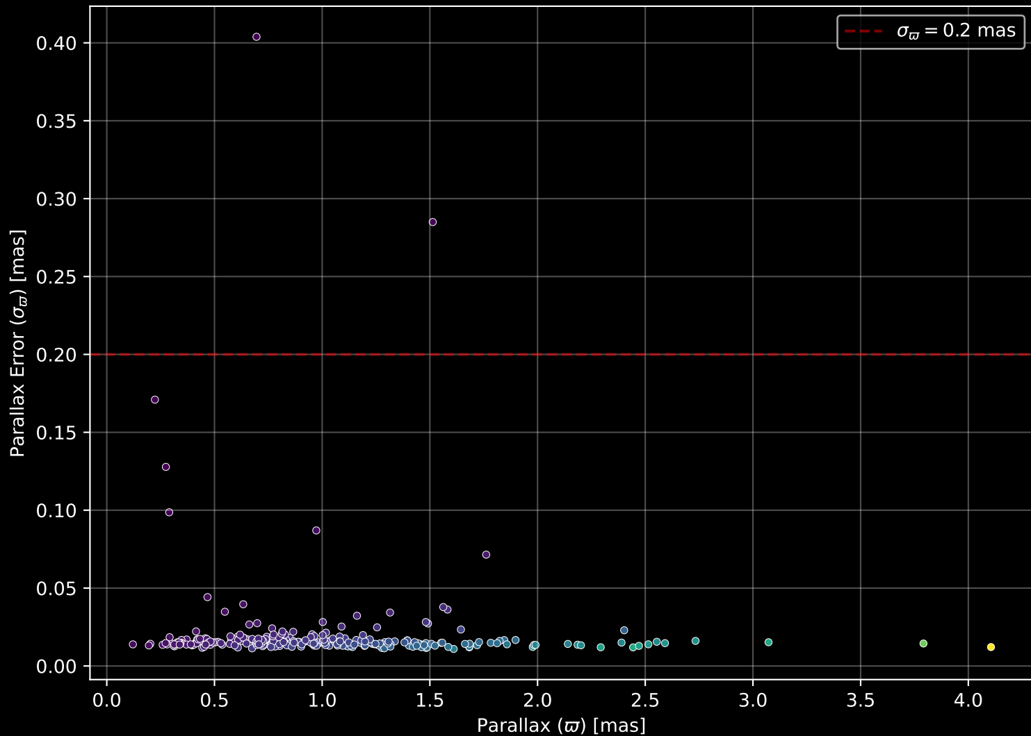
GALAH DR4 Field: [8823] Parallax Quality (n= 258)
