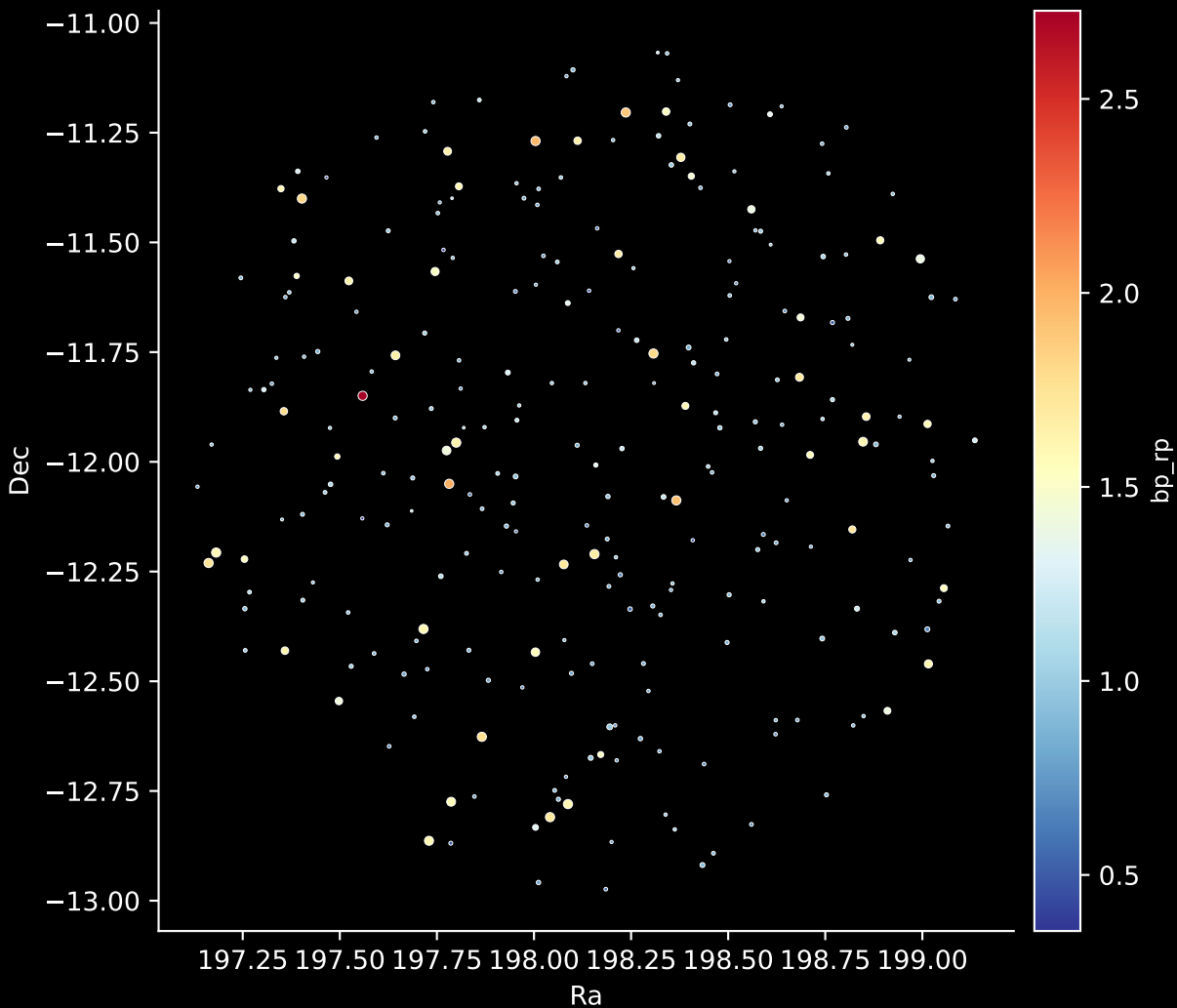
GALAH DR4 Field: [8823] Stars: 258
